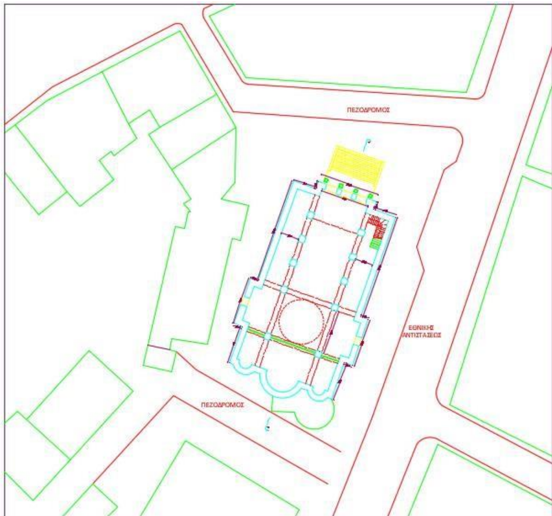
Κάτοψη του Ιερού Ναού
